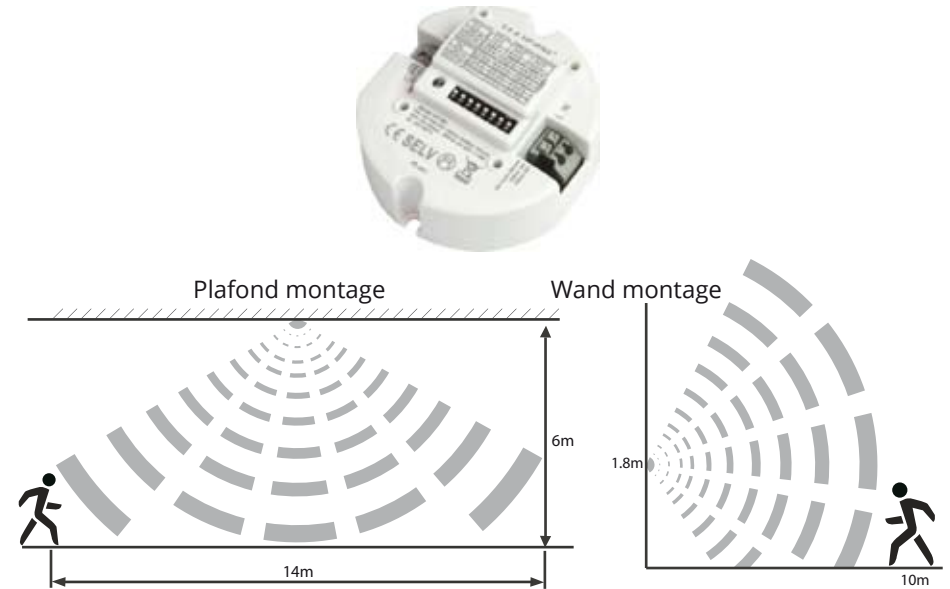
De detectiesensor heeft een circulair bereik, de detectiezone kan worden vergroot of verkleind afhankelijk van de situatie en installatie hoogte.
